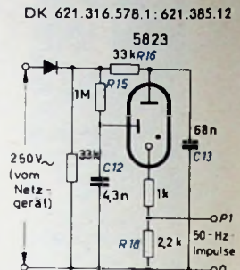
Bild 2. Schaltung des Netzgerätes A
