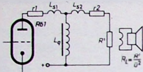
Bild 1. Eintakt-Ausgangsübertrager, Ersatzschema
