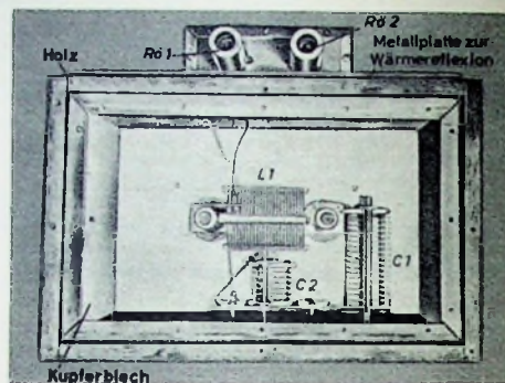
Bild 5. Blick von oben in den geöffneten Oszillator. Der Resonanzkreis befindet sich in einem mit Kupferblech ausgekleideten Holzkasten, während alle anderen Teile im Metallgehäuse an der Außenseite des Holzkastens untergebracht sind
