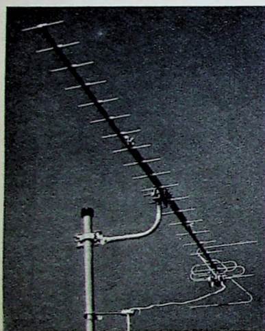
Die UHF-Super-Breitbandantenne „DFA 1 LM 51“ von fuba läßt sich sehr gut zusammenklappen
