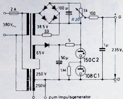
Bild 2. Schaltung des Netzgerätes A
