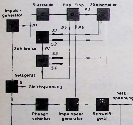
Bild 1. Blockschema eines elektronisch gesteuerten Ignitron-Schweißbäckers
