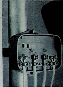
Antennenweiche von Hirschmann mit Schnellspannklemmen
