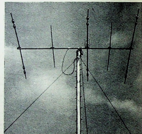
Element X [mm] Y [mm] Z [mm] Gesamtlänge [mm] Direktor II 640 570 890 7400 Direktor I 4680 Strahler 880 550 930 7920 Reflektor I 5200 Reflektor II 1005 650 960 8430
