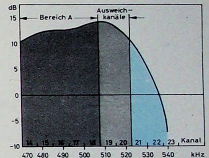
Starker Abfall des Gewinns einer UHF-Kanalgruppen-Antenne außerhalb ihres Bereiches (nach fuba)
