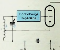
Bild 3. Die Realisierung der isolierenden hochohmigen Impedanz durch einen Kathodenverstärker
