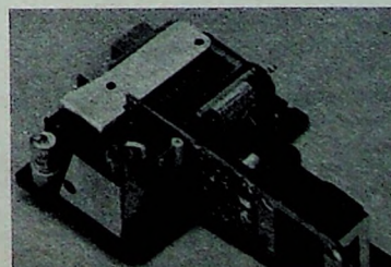
Chassis des Senders. Rechts: Transistor-Gleichspannungswandler; links: Oszillatorschaltung; oben: Röhre, Antennenkreisschaltung und Antennen-Verlängerungsspule
