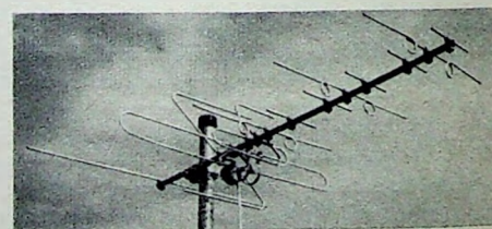
„Comбина“, Mehrbandantenne (Bänder III ... V) von Kathrein; für UHF sind 13 Elemente wirksam
