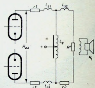
Bild 2. Ersatzschema eines Gegentakt-Ausgangsübertragers (für \bar{u} = 1 umgerechnet)
